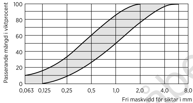
FIGUR AMA FS/1. KORNKURVA FÖR BALLAST TILL MURBRUK.
