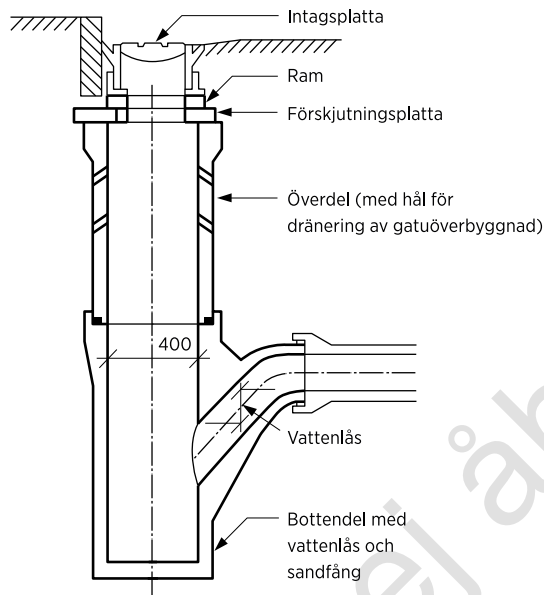
Exempel på dagvattenbrunn av betong med vattenlås och sandfång
