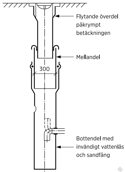
Exempel på dränvattenbrunn av plast med invändigt vattenlås och sandfång, vattenlåset utformat för att möjliggöra renspolning av anslutande dränledning
