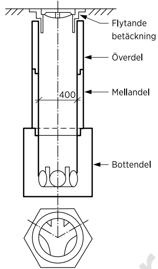
Exempel på tillsynsbrunn av betong
