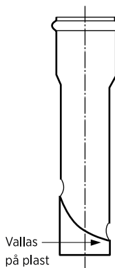
Exempel på bottendel till dränvattenbrunn av plast, utan vattenlås, utan sandfång
