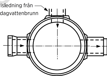
Exempel på nedstigningsbrunn av betong, med sandfång
