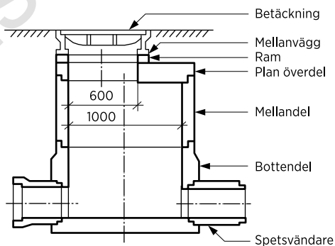
Exempel på nedstigningsbrunn av betong. Lågbyggd brunn med plan överdel
