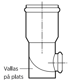
Exempel på bottendel till dagvattenbrunn av plast, utan vattenlås, utan sandfång
