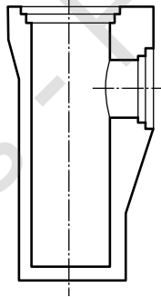
Exempel på bottendel till dagvattenbrunn av betong utan vattenlås, med sandfång
