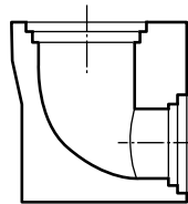
Exempel på bottendel till dagvattenbrunn av betong utan vattenlås, utan sandfång
