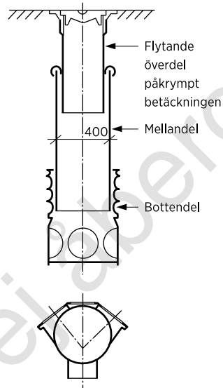
Exempel på tillsynsbrunn av plast. Tillsynsbrunnar av plast förekommer även i dimension 315
